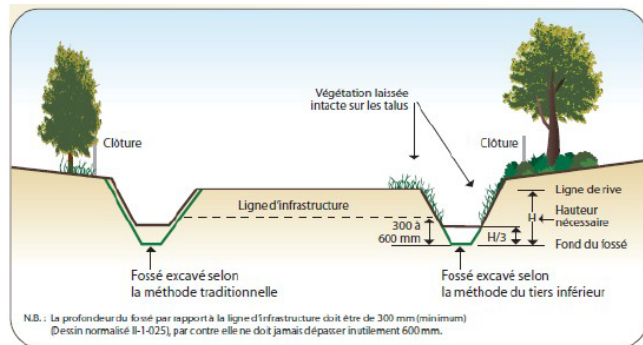
Schéma représentatif d'une des techniques alternatives pour l'entretien des bords de routes: Comparaison entre la méthode traditionnelle et celle du tiers inférieur
